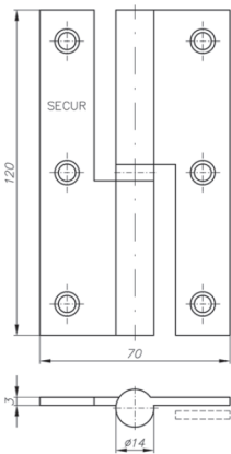
Zawias prawy
