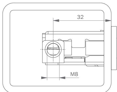
SEZ. A-A
