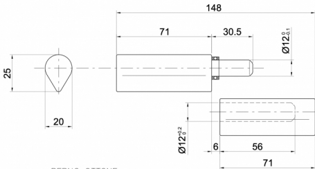
PERNO OTTONE CUSCINETTO ZINCATO
