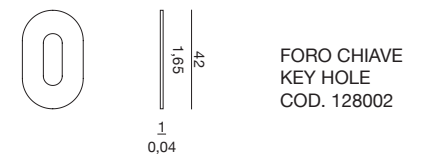
A. BOCCHETTA SLIM / SLIM ESCUTCHEON
