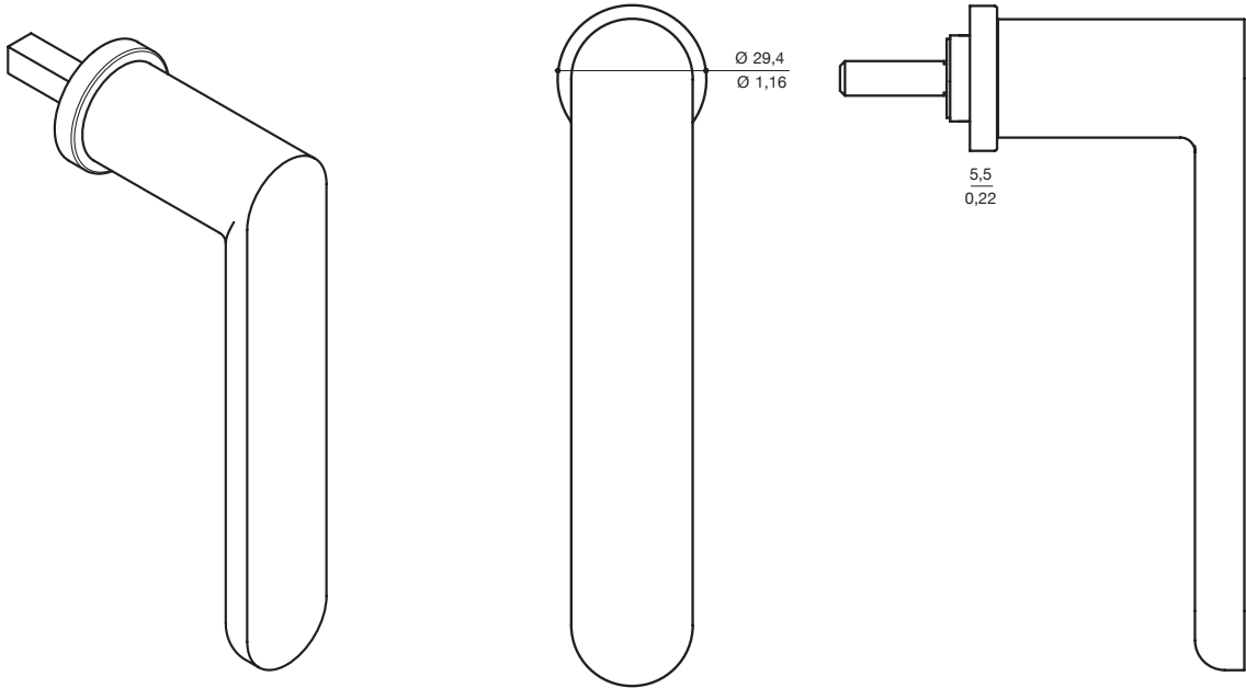
QUADRO / SPINDLE 7 MM / 0,27 INCH
