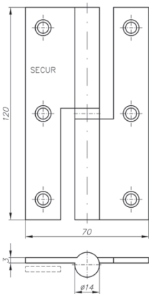
Zawias lewy
