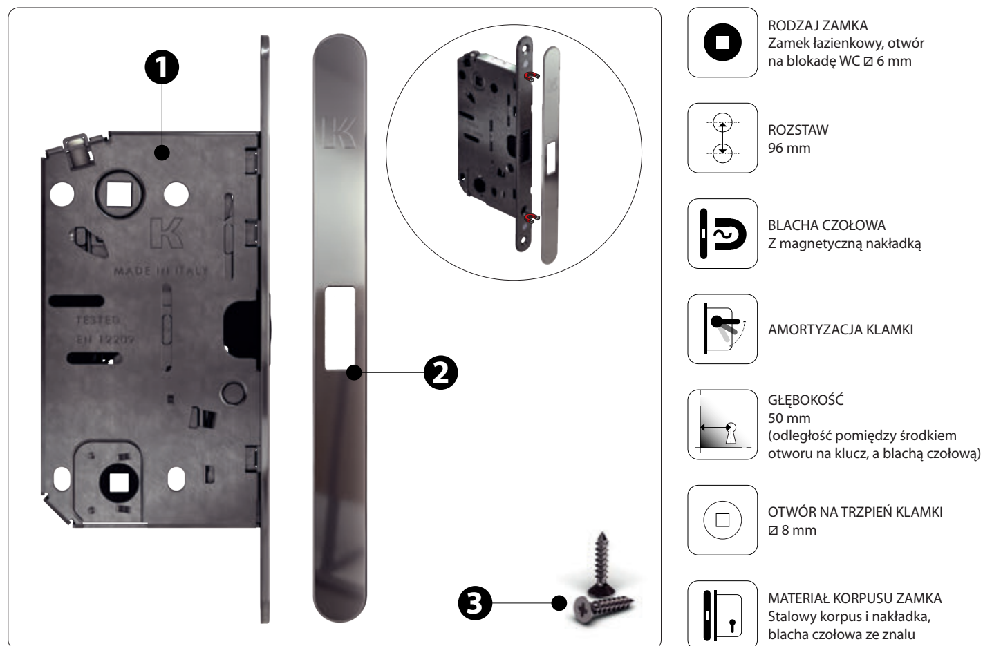
RYSUNKI TECHNICZNE
