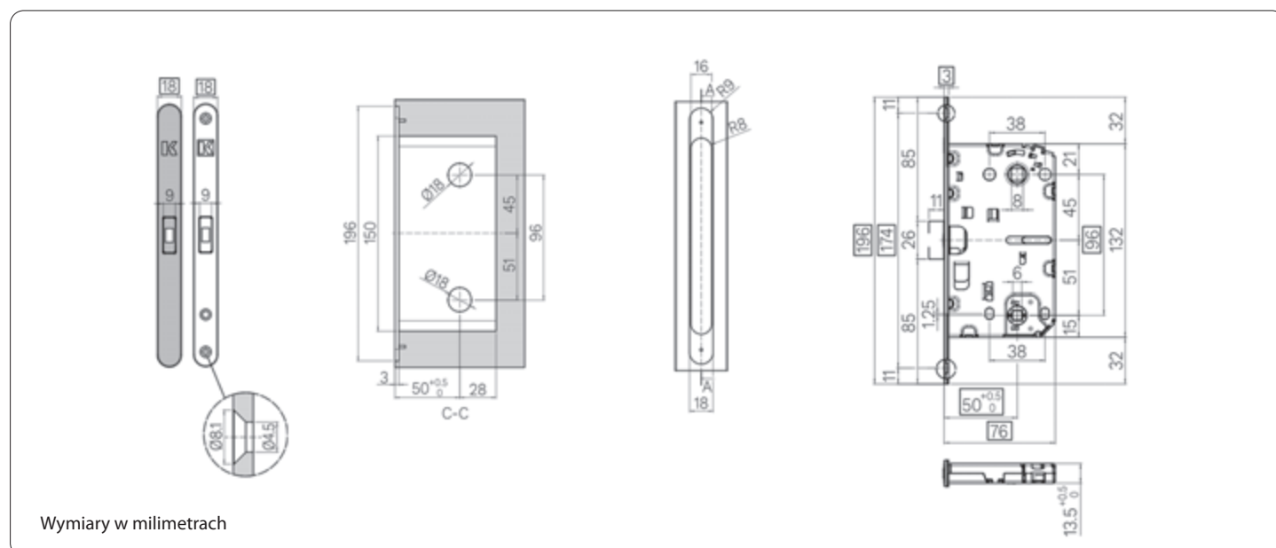
RYSUNKI TECHNICZNE
