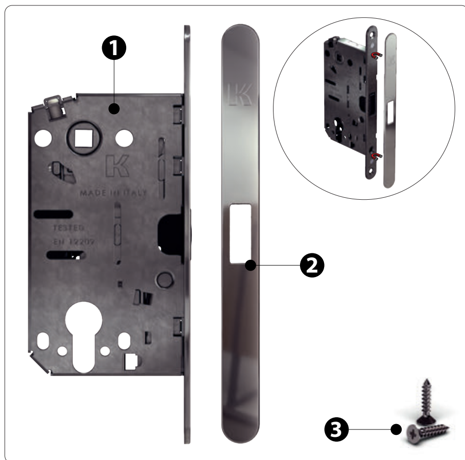
RYSUNKI TECHNICZNE
