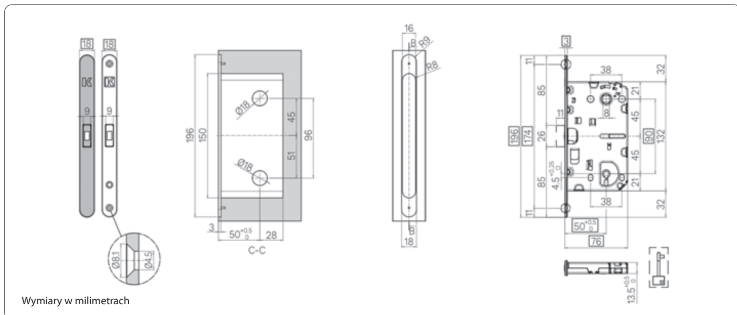
RYSUNKI TECHNICZNE
