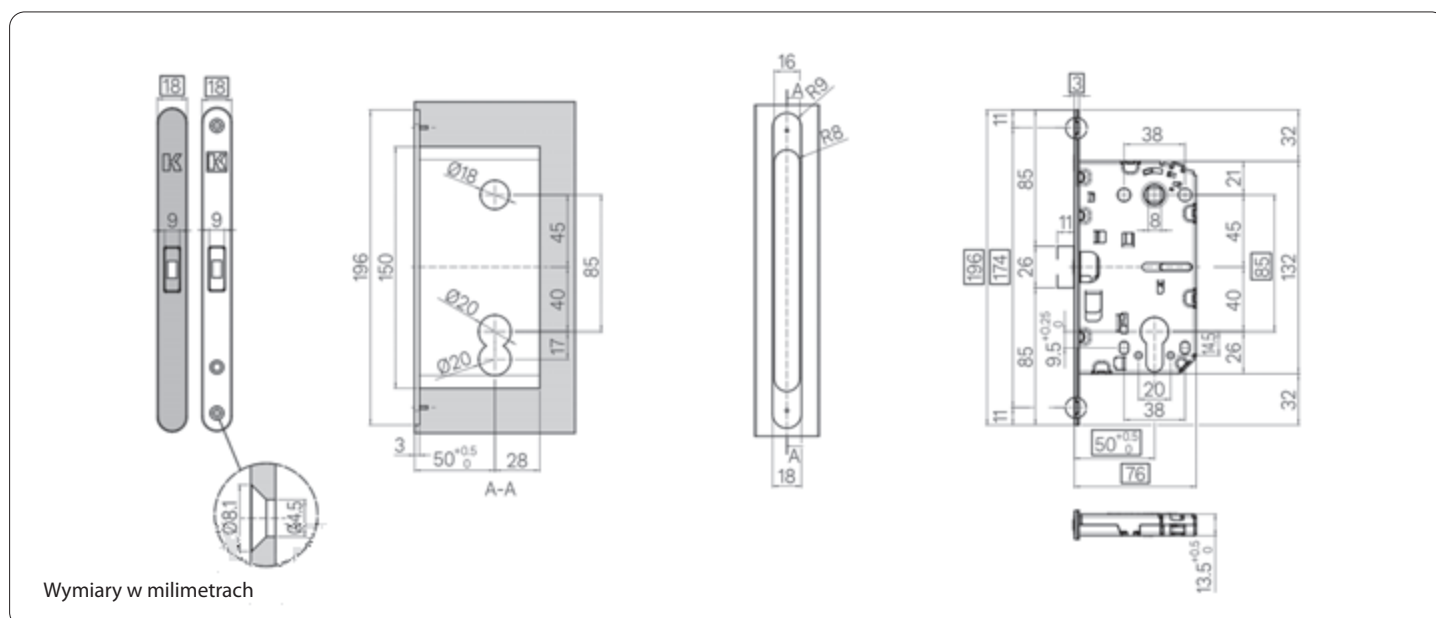
RYSUNKI TECHNICZNE
